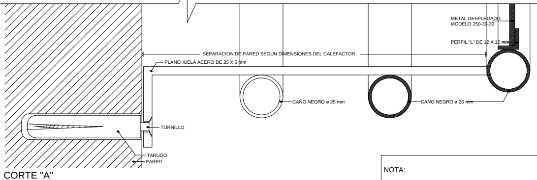
DETALLE DE PLANCHUELA FIJADORA EN PARED
