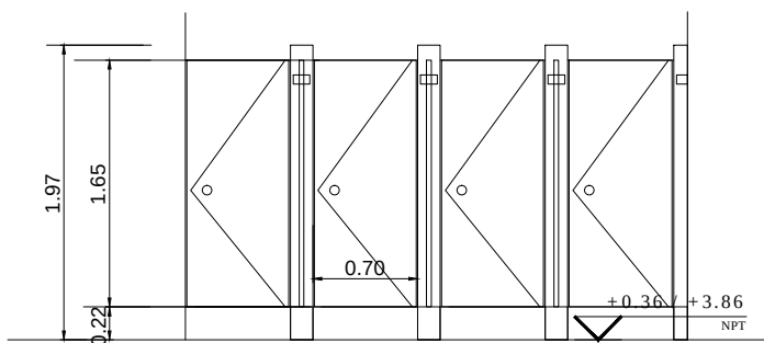
Vista Puerta
