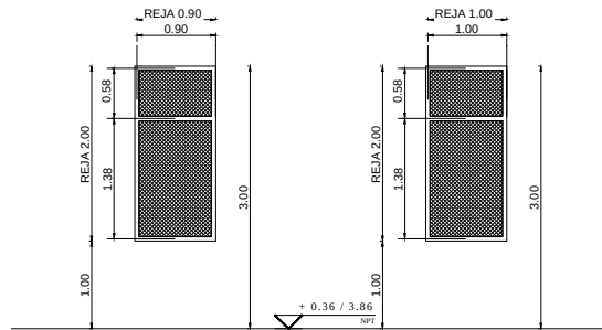
Vista Reja
