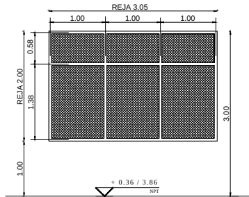
Vista Reja
