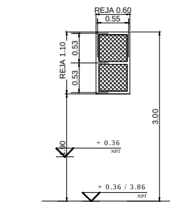
Vista Reja
