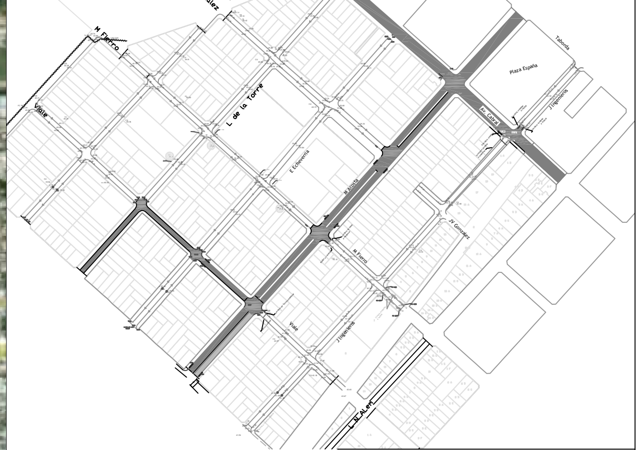
— Cordon Cuneta Proyectado ← Ecurrimiento Superficial
