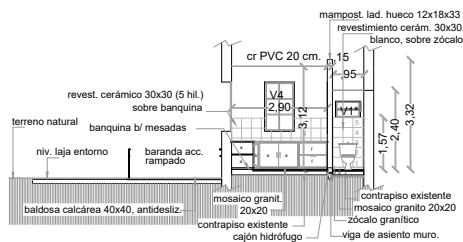
CORTE C-C
