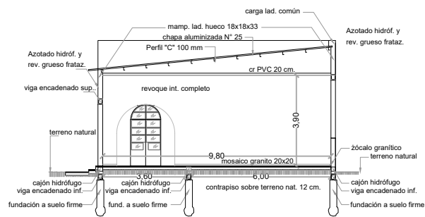
CORTE D-D
