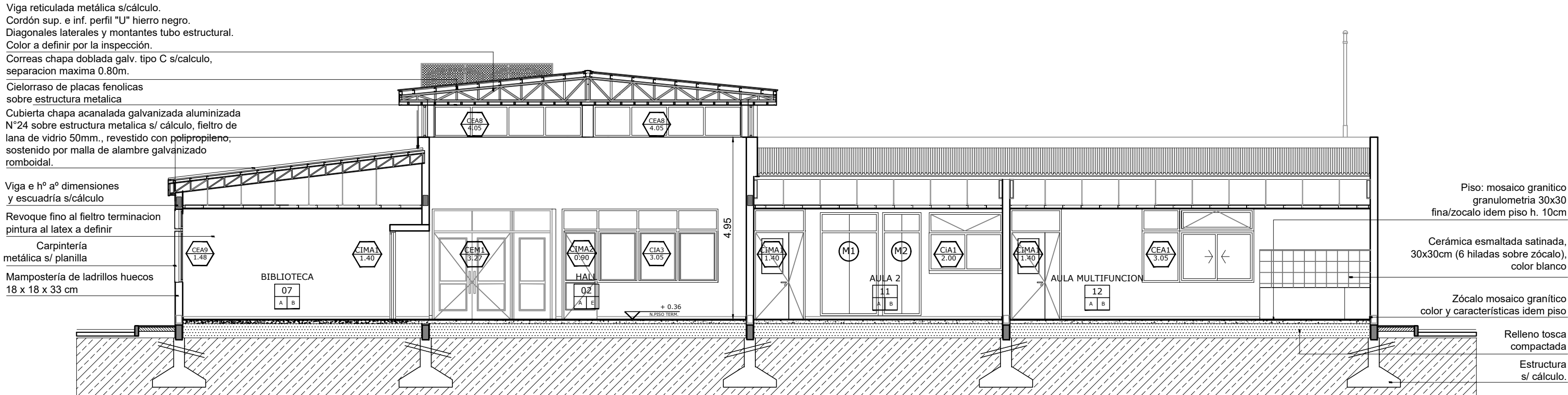
CORTE B-B
